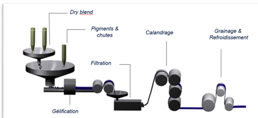
Figure 1 : Processus de Calandrage
